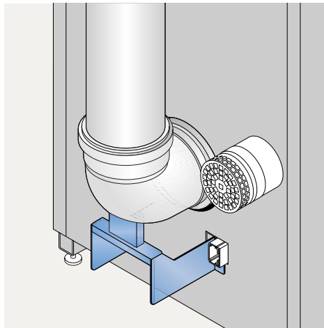
Die serienmäßige Stützkonsolle erleichtert die Montage der Abgasleitung (WTC-GB 120-300)
