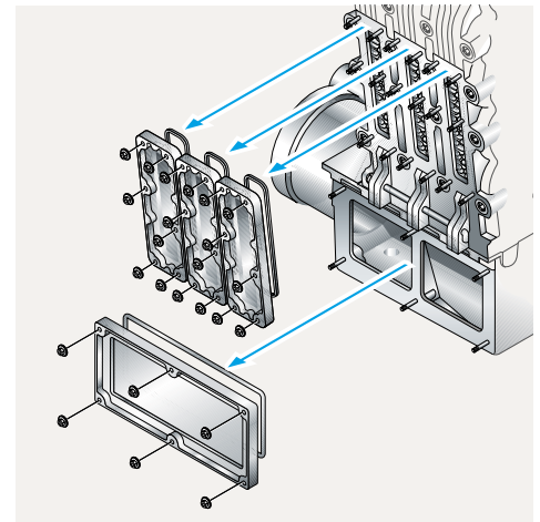
Der Wärmetauscher ist über mehrere große Revisionsöffnungen gut zugänglich
