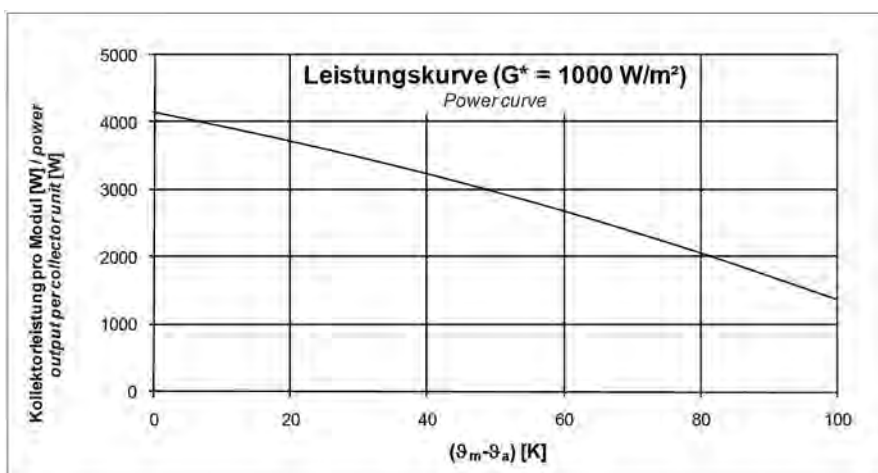
Kurve für AS 6 Großflächenkollektor
